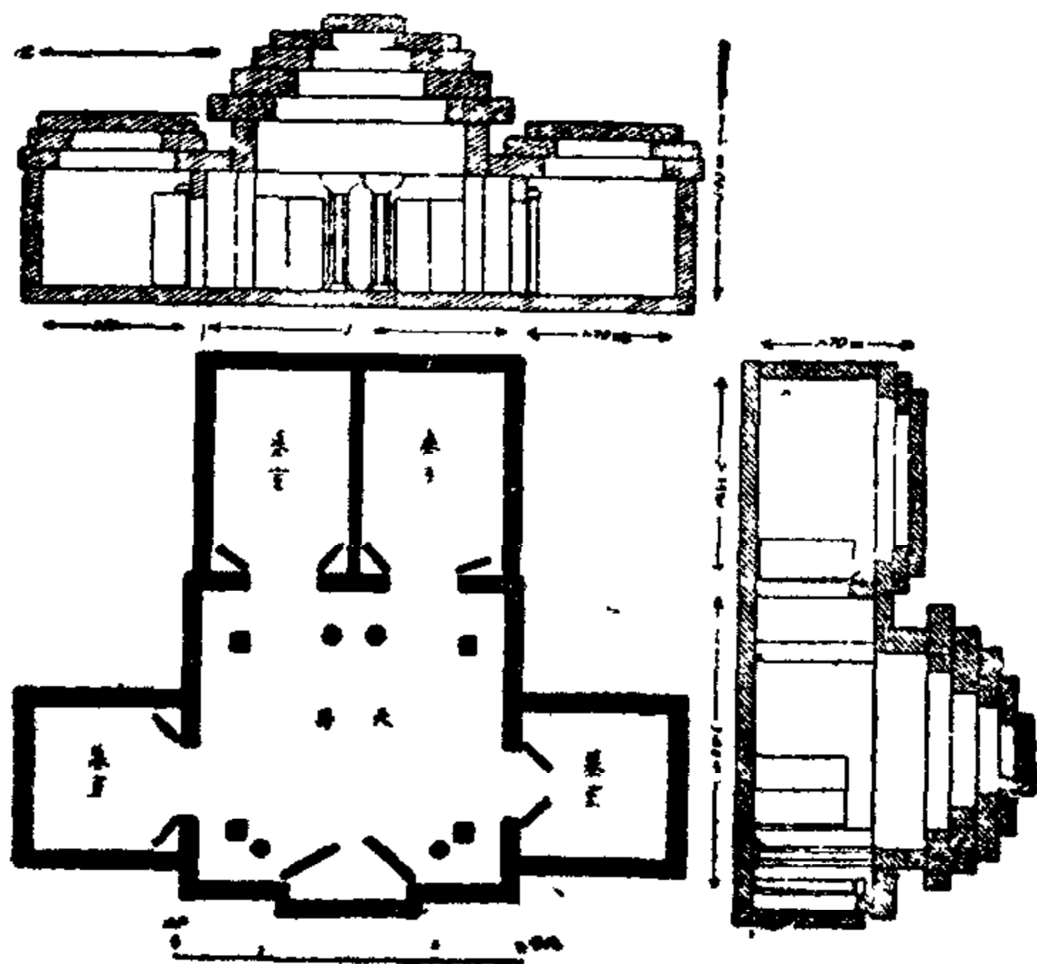
滕縣宋代墓葬實測圖
